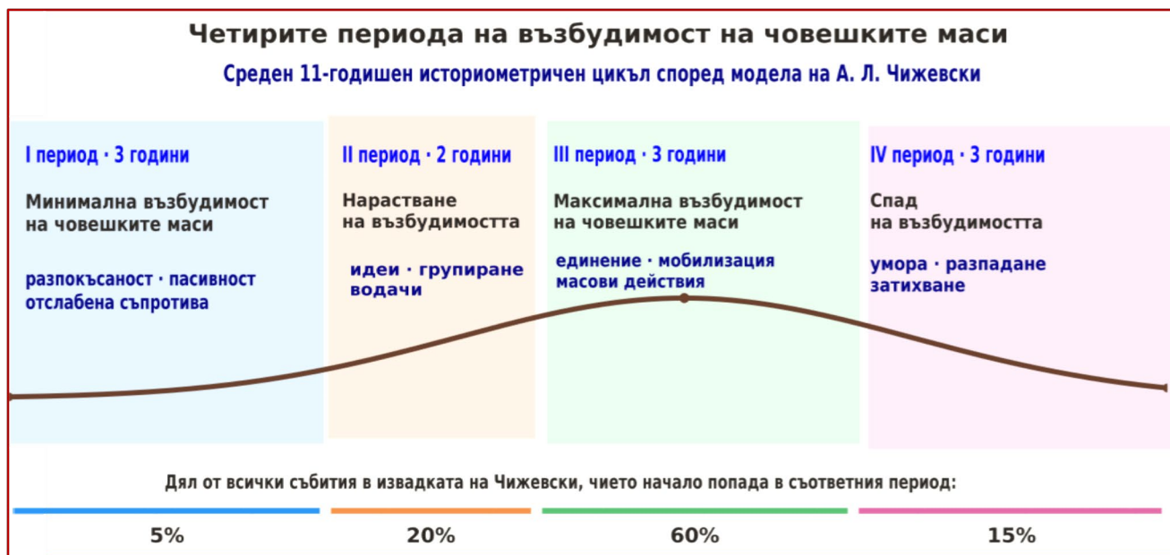
Фиг. 1 Периоди на 11-годишния цикъл по Чижевски
